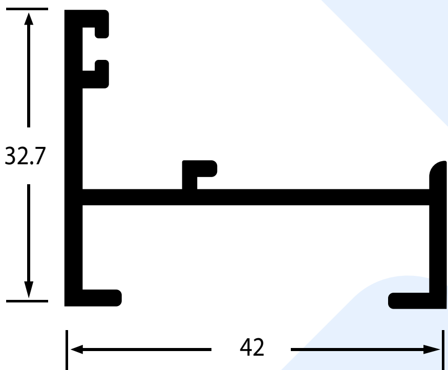
Marco
