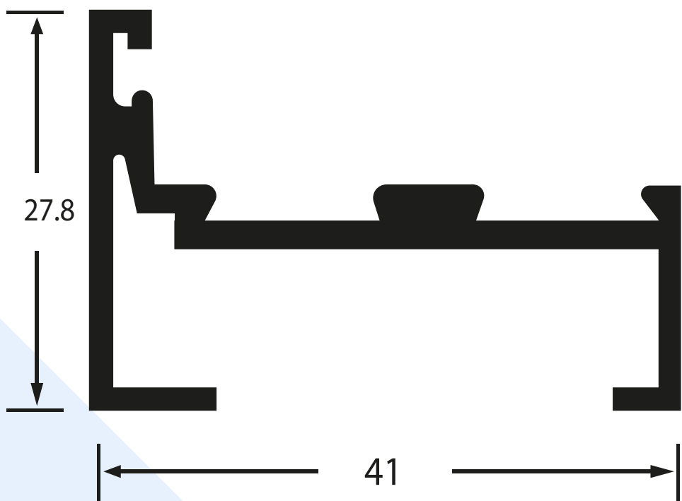
Marco
