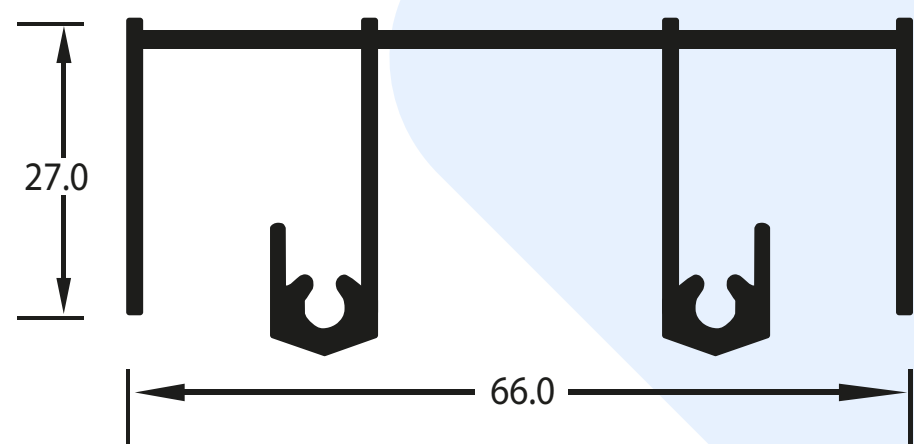
Doble riel superior
