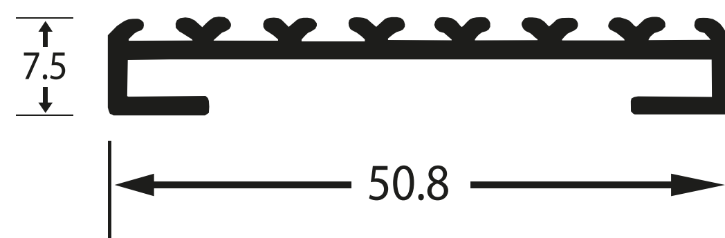
Cortaviento
