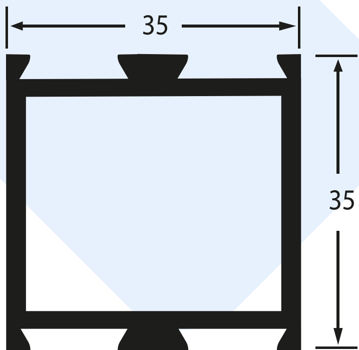
Bastidor
