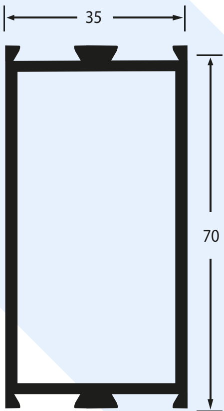
Bastidor
