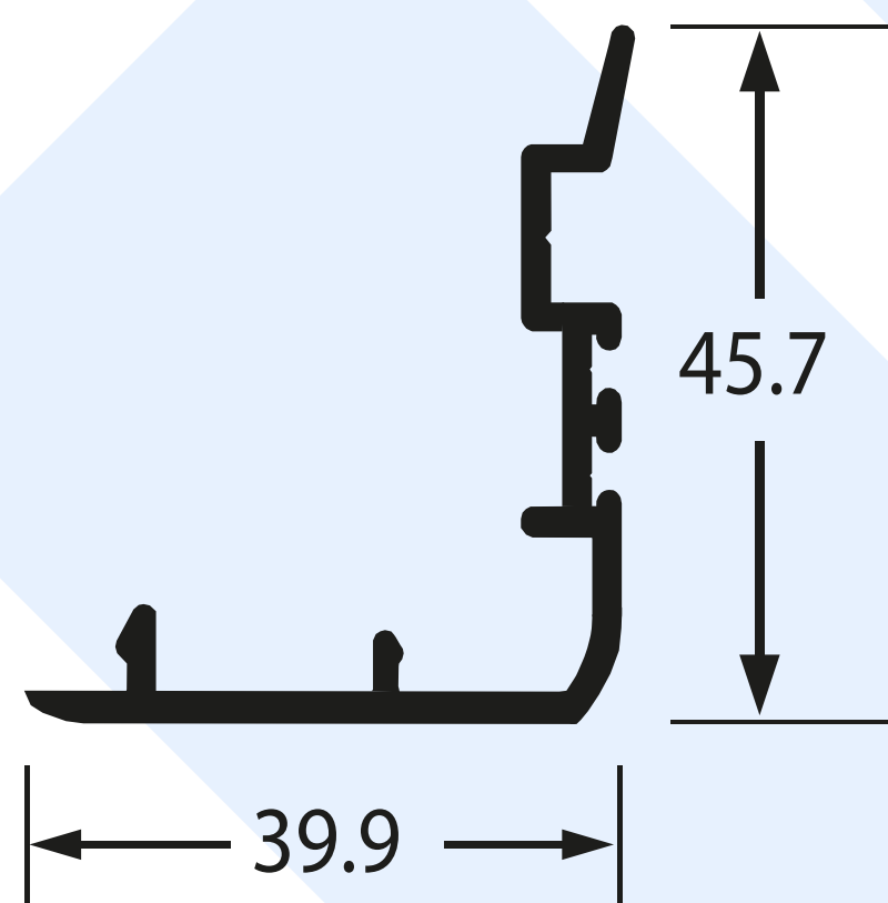
Traslape de hoja
