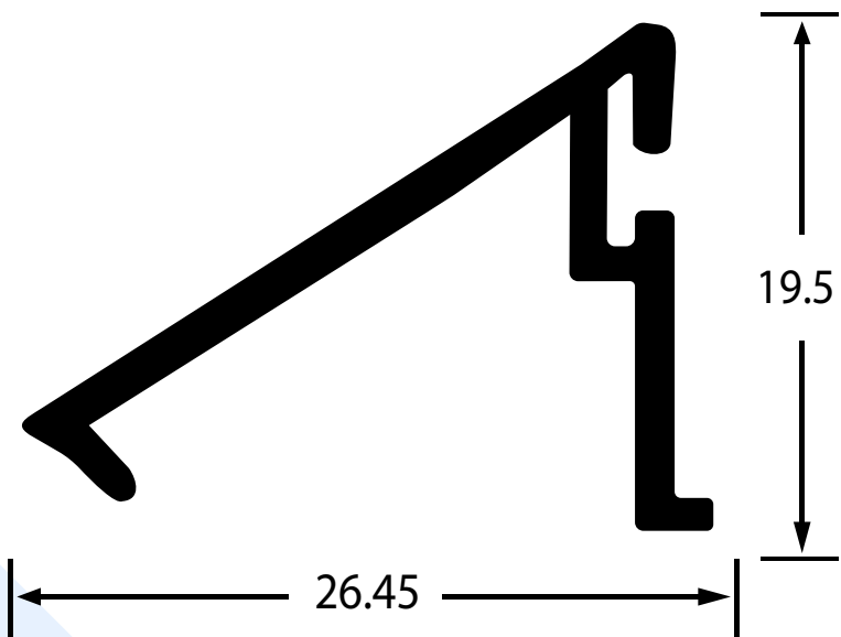
Junquillo
