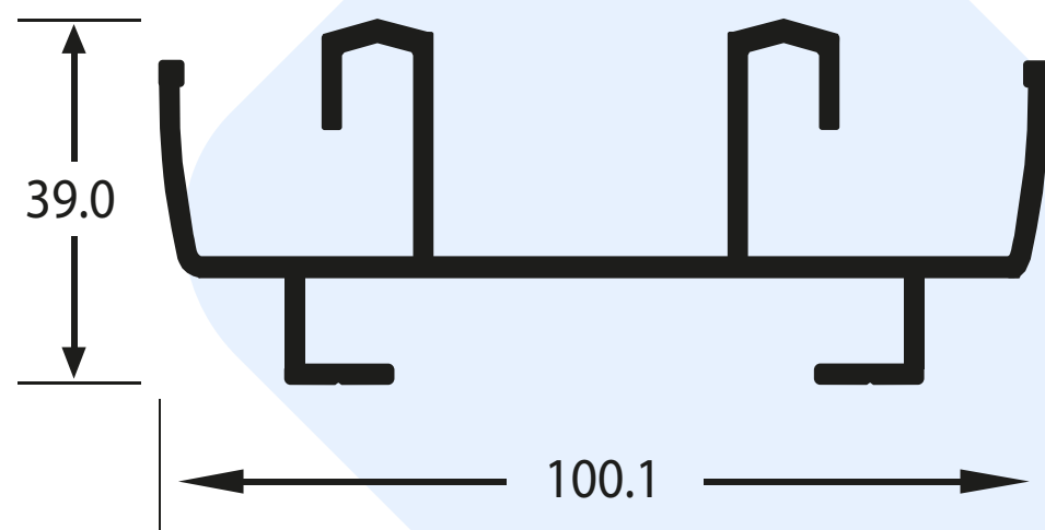
Marco doble corrediza
