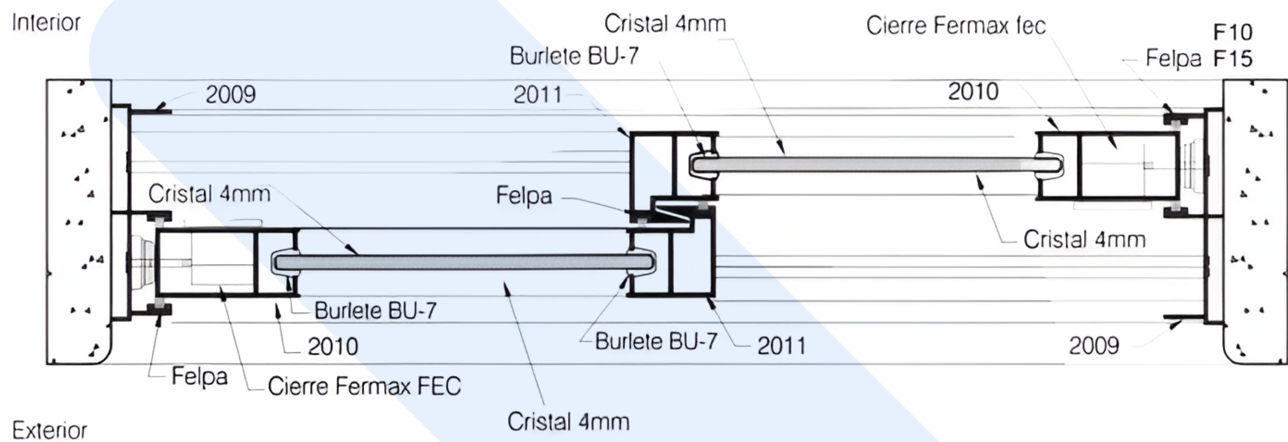
Vista horizontal
