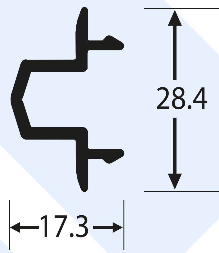
Adaptador de hoja
