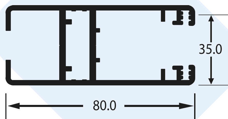
Marco de hoja
