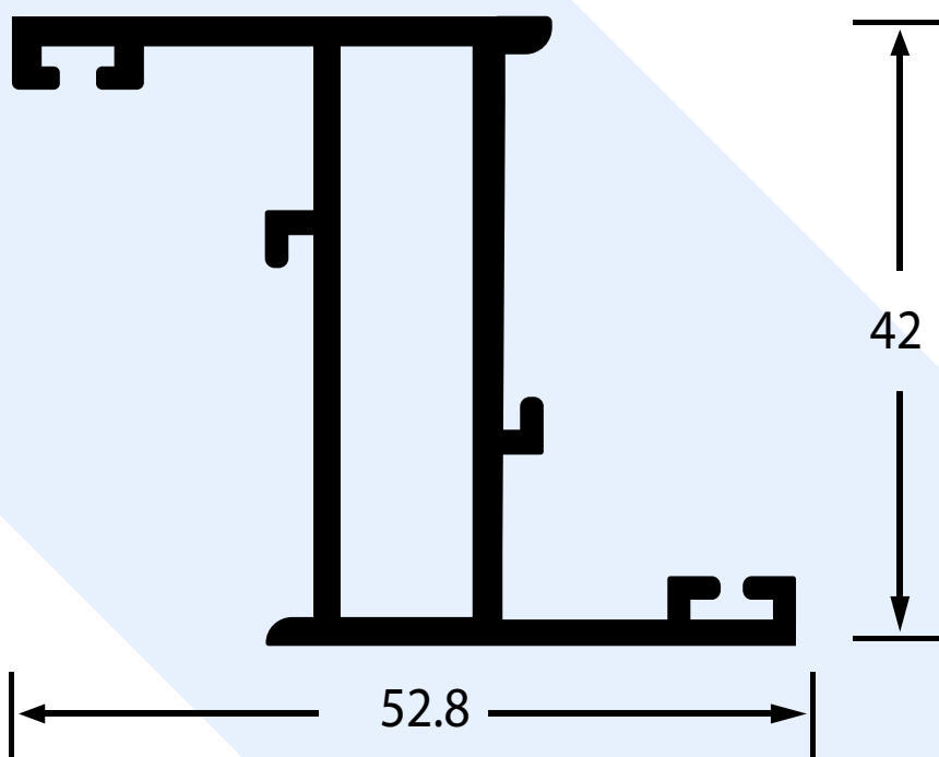
Marco nave
