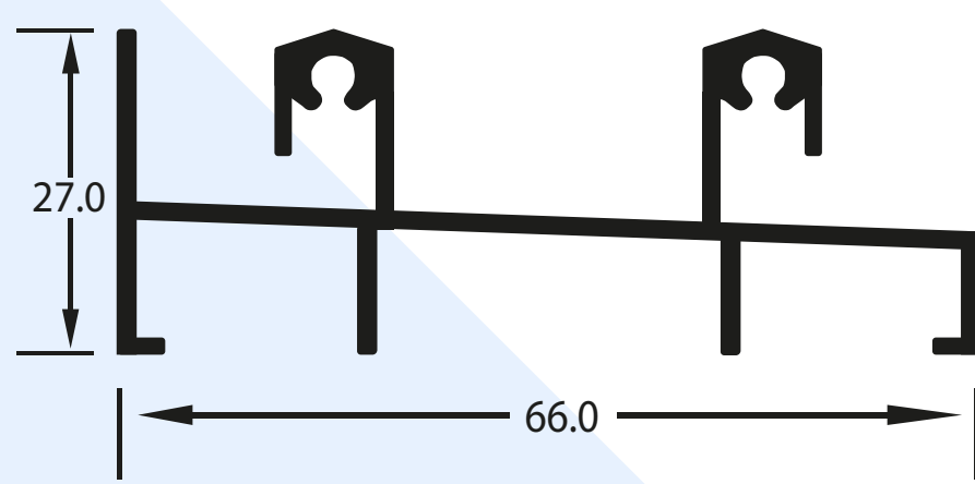
Doble riel inferior
